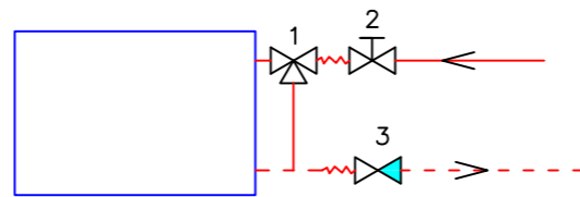
Šema spajanja ventilokonvektora
