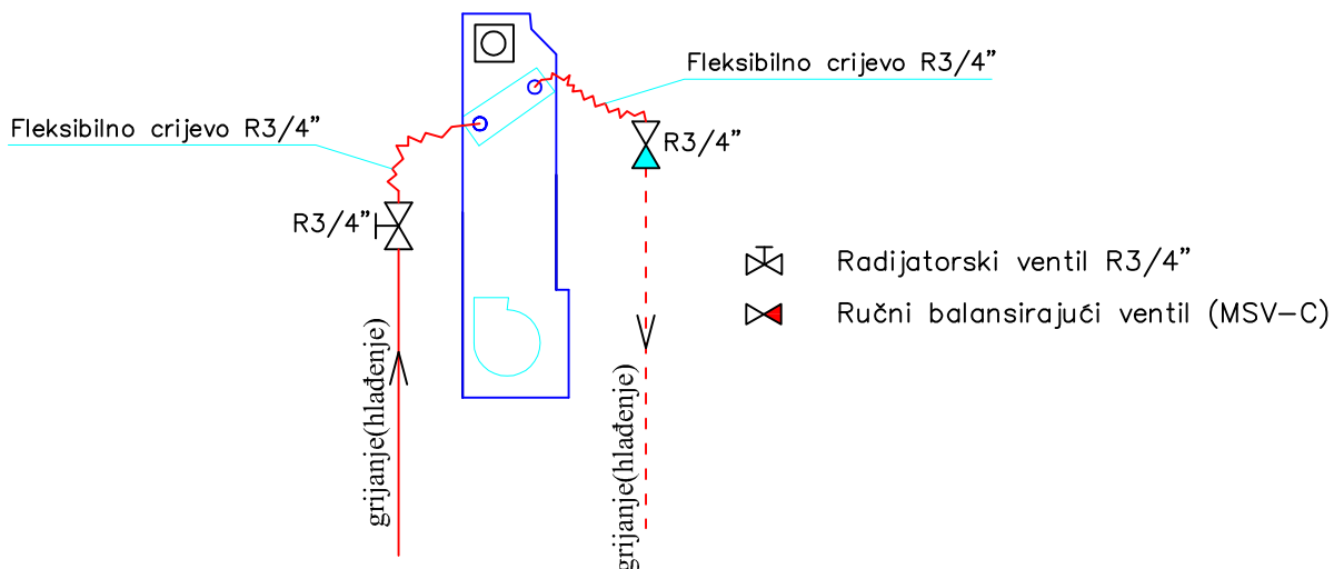
Šema parapetnog ventilokonvektora
