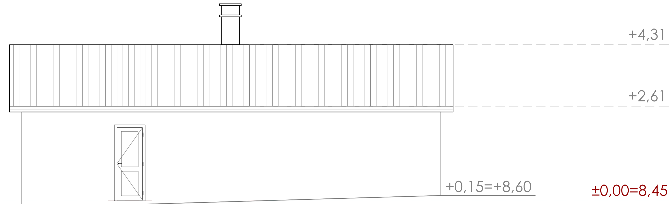
SJEVERNO PROČELJE
